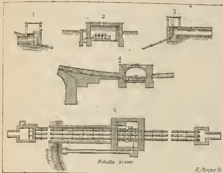
Fig. 1. Detalles del sifón de los Gruidi
